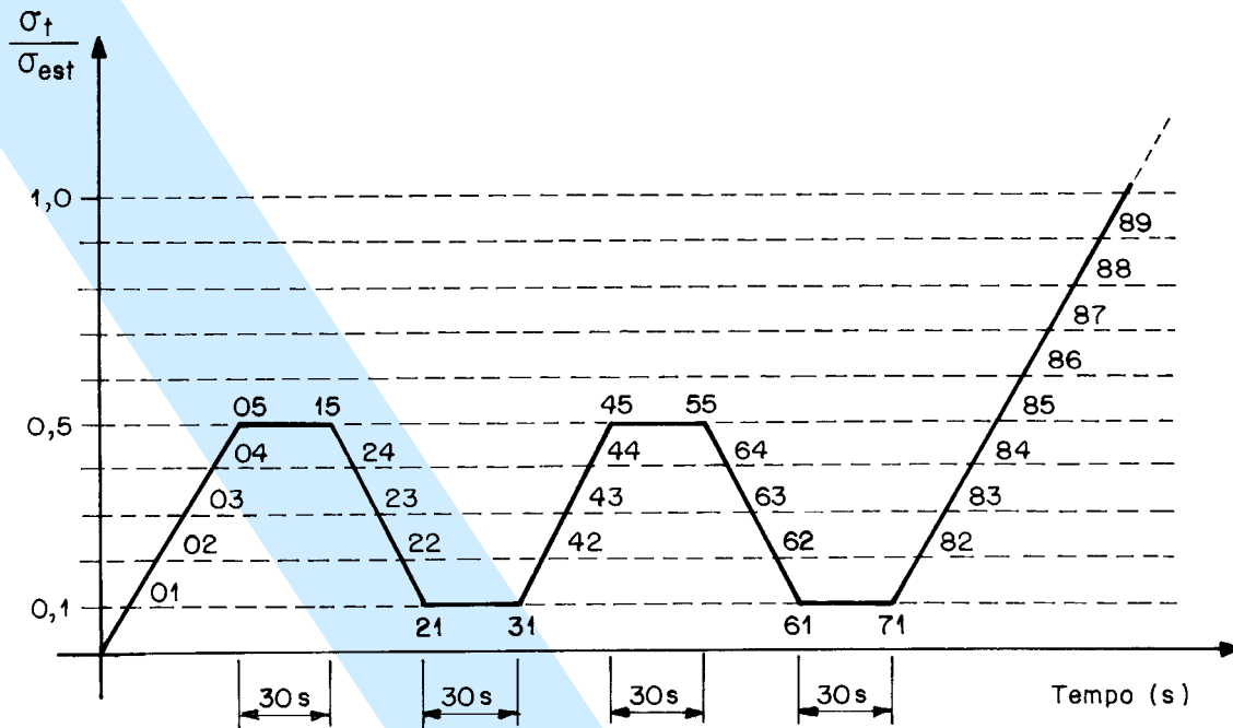
Figura B.11 - Diagrama de carregamento para determinação da rigidez da madeira à tração
